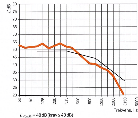
Figur 1. Ljudmätningar för bjälklagets ljudisolering i ett tvåvånings provhus när det var "färdigutvecklat", det vill säga efter modifieringar för att kunna uppfylla ljudklass A, 2008.
